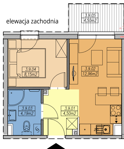
RZUT MIESZKANIA skala 1:100
