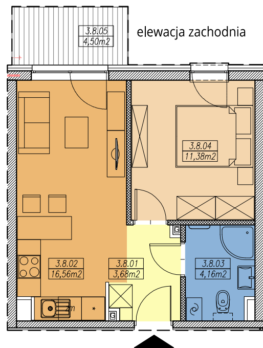
RZUT MIESZKANIA skala 1:100
