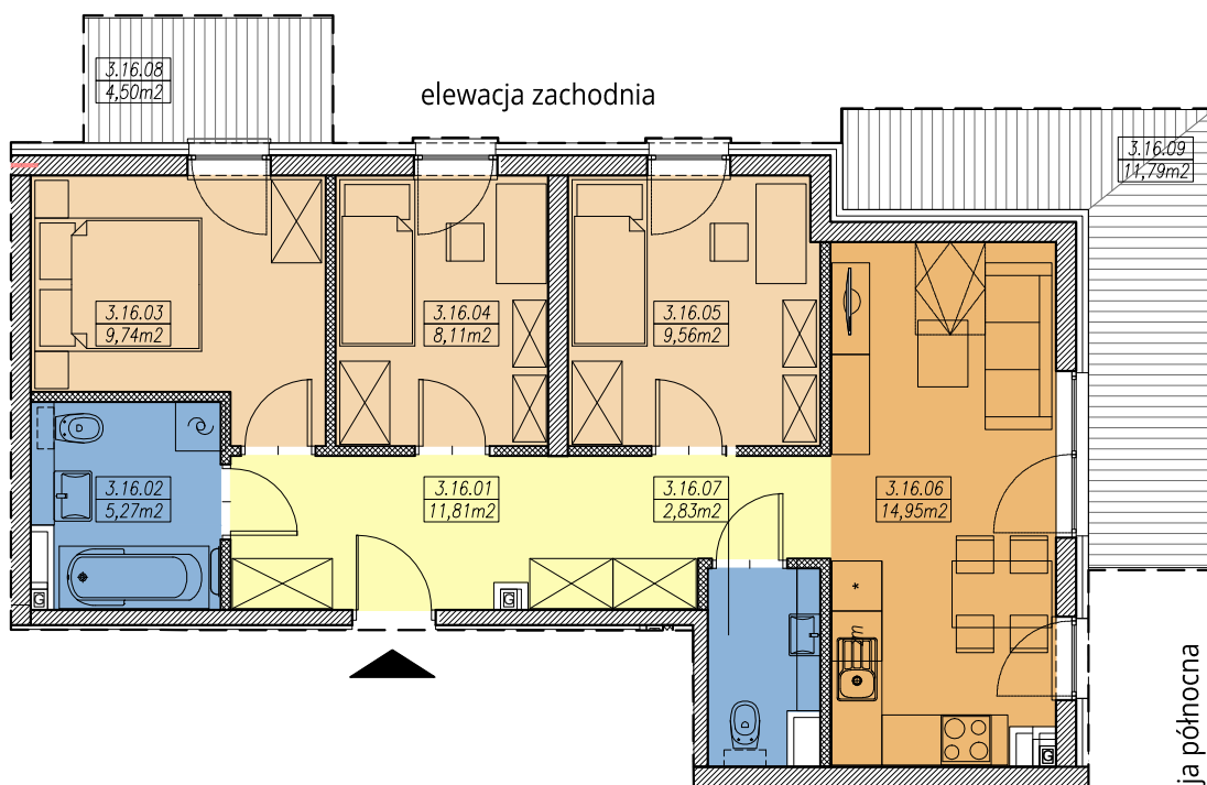
RZUT MIESZKANIA skala 1:100
