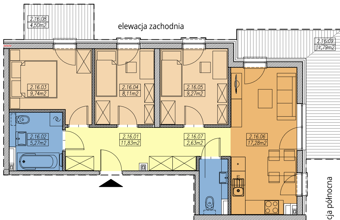
RZUT MIESZKANIA skala 1:100
